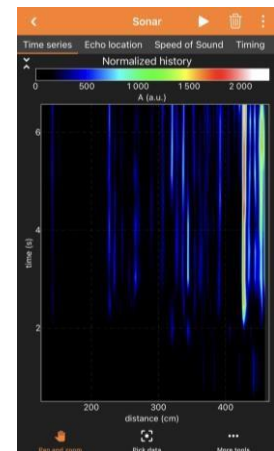
Рис.6. Вимірювання відстані через відлуння та швидкість звуку
