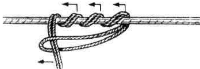
Мал. 6.19. Вузол «австрійський схоплюючий»
