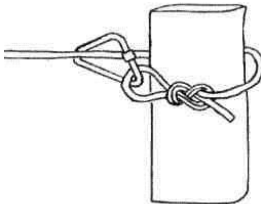
Мал. 6.13. Карабінна удавка
