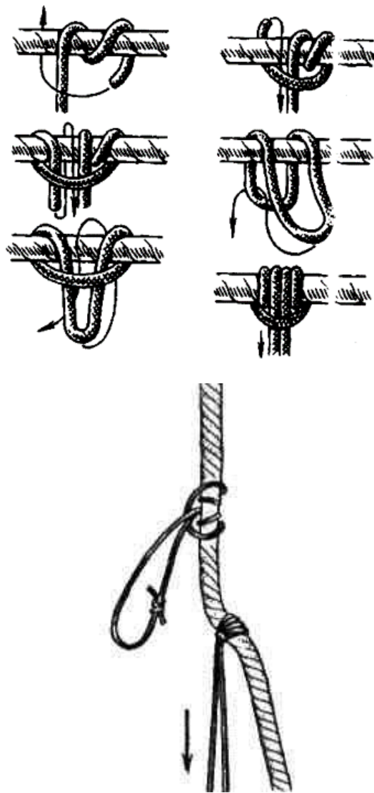
Мал. 6.17. Вузол «схоплюючий»
