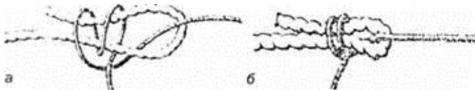
Мал. 6.6. Брамшкотовий вузол: а – в'язання вузла; б – навантажений вузол
